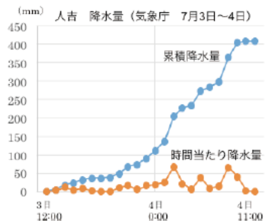
図1 人吉 降水量の記録（気象庁）
