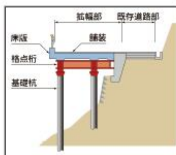
図3 メタルロード標準断面図
